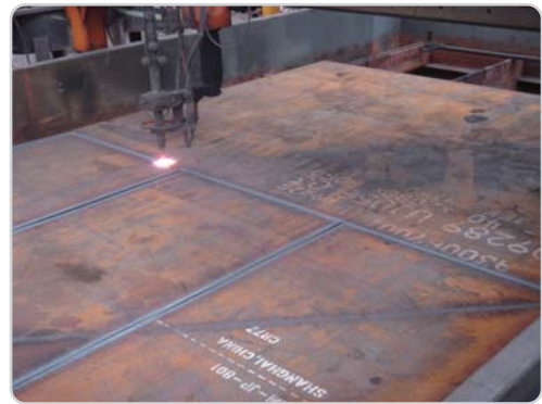
数控火焰切割
